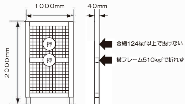
金網中央部の破壊点：2520N 横フレームの破壊点：8680N
